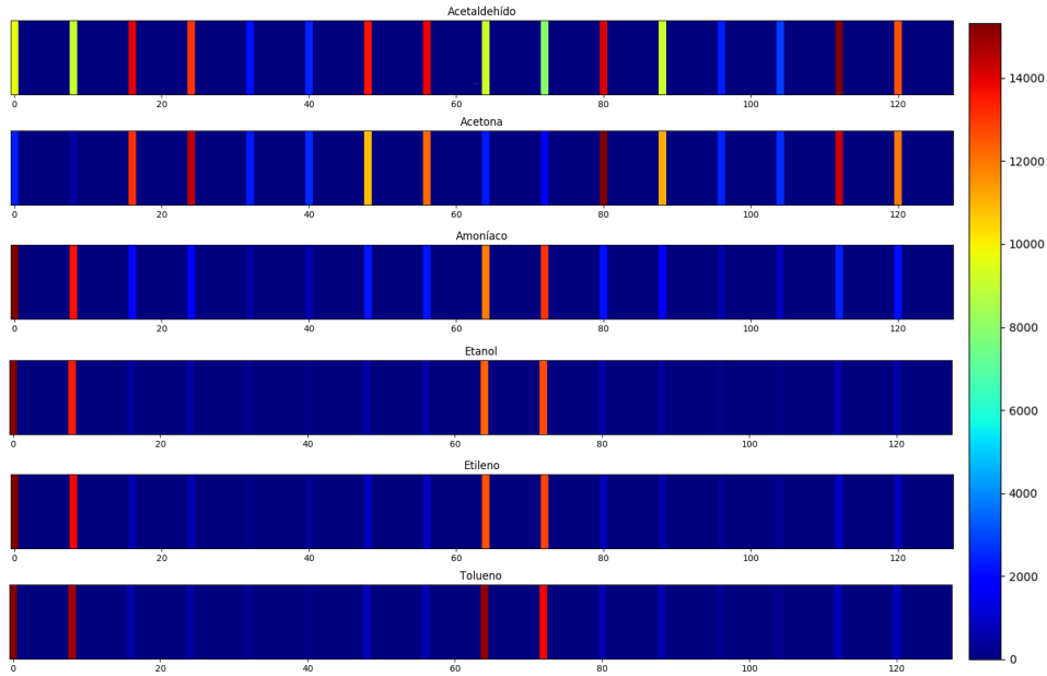
Figura 3.6: Vectores de 128 características correspondientes a cada uno de los seis posibles odorantes a una concentración de 50ppmv. El conjunto de datos han sido obtenidos de [68]
