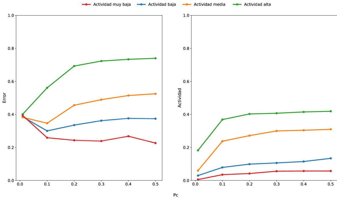
Figura 4.6: Error de clasificación y activación media de las neuronas KCs promediado para los patrones MNIST. Los resultados que se muestran son el promedio de 10 simulaciones.
