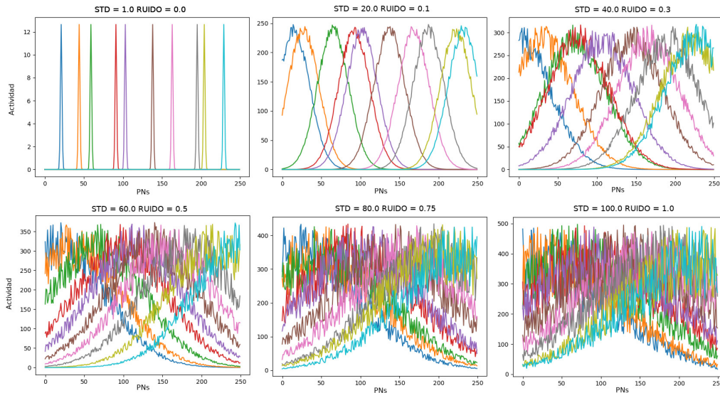
Figura 3.4: Patrones gaussianos de complejidad creciente de izquierda a derecha y de arriba a abajo, según el solapamiento de las clases (debido a la desviación estándar de las gaussianas, STD) y el nivel de ruido. El eje X se corresponde con las 250 neuronas PNs y el eje Y con la activación de cada neurona. En cada uno de los gráficos se muestra un ejemplo de patrón por cada una de las 10 clases existentes.
