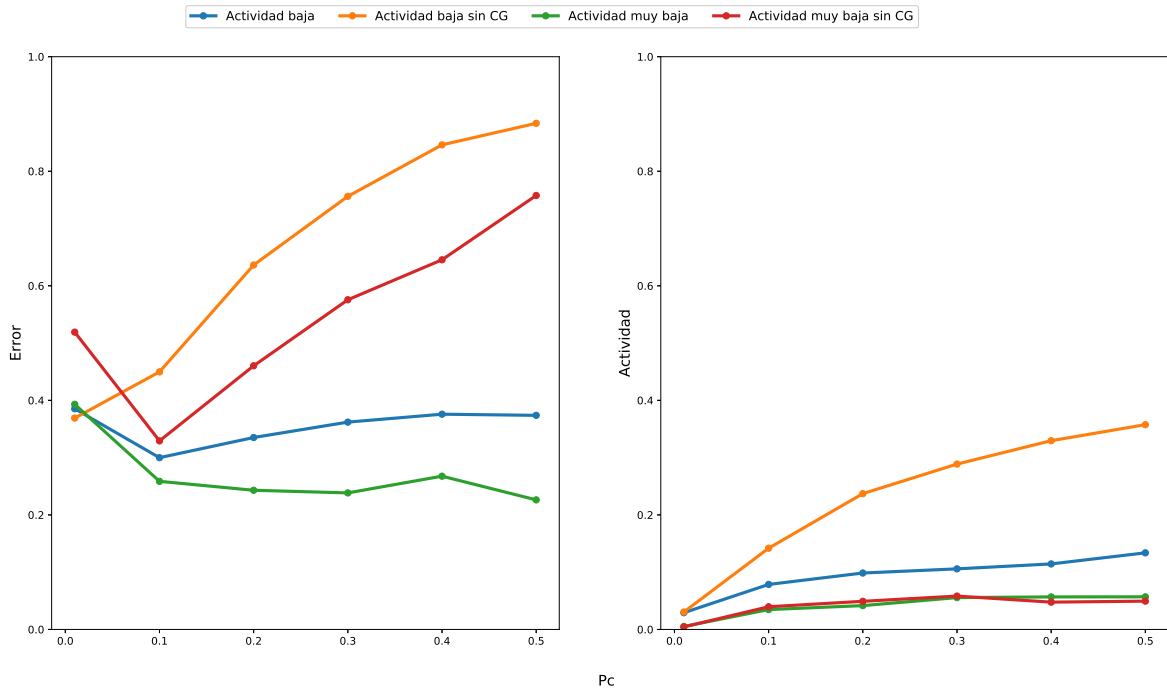
Figura 4.9: Comparación entre el error de clasificación y el nivel de actividad obtenido utilizando o no el mecanismo de control de ganancia. Las diez simulaciones por cada punto se han realizado para el nivel bajo y muy bajo de actividad, al ser los que obtienen mejores resultados, y todos los valores de p_c considerados.
