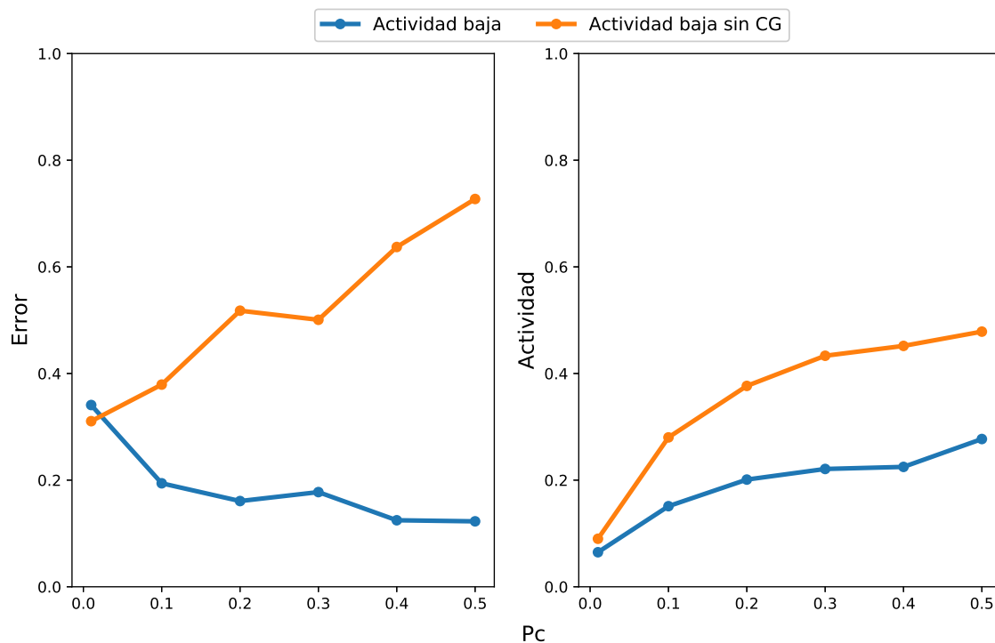
Figura 4.13: Resultados obtenidos para el nivel bajo de actividad con los diferentes valores de p_c con y sin incluir el control de ganancia. El modelo se ha entrenado con los patrones del conjunto de olores B_1 y se ha evaluado con el conjunto B_2 .
