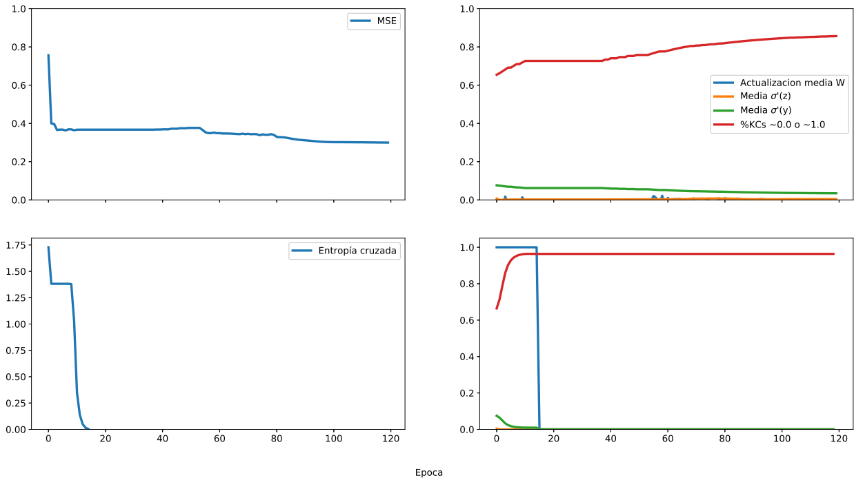
Figura 3.3: Comparativa entre el uso del MSE (fila superior) como función de coste y la entropía cruzada (fila inferior). En la parte derecha de la figura se muestra la evolución del MSE y de la entropía cruzada en función del número de épocas, mientras en la parte izquierda se muestran la evolución de diferentes parámetros y medidas del sisema. Entre estas medidas destacan el valor de actualización de los pesos en color azul y una medida de la convergencia de la red en rojo que se corresponde con el porcentaje de KCs de la capa oculta que poseen valores medios de activación cercanos a 0 o a 1.
