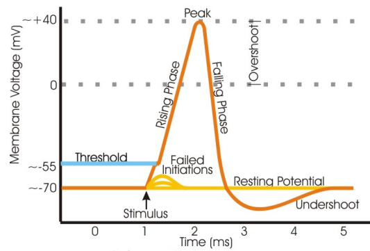
Figura 2.1: Potencial en la membrana frente al tiempo durante un disparo neuronal. Cuando el potencial de membrana supera el valor del umbral, se produce el disparo neuronal. Los incrementos del potencial que no alcanzan el valor del umbral no producen disparos y regresan al potencial de reposo con el tiempo. Figura realizada por Synaptitude en en.wikipedia [GFDL ( http://www.gnu.org/copyleft/fdl.html ) o CC-BY-SA-3.0 ( http://creativecommons.org/licenses/by-sa/3.0/ )], vía Wikimedia Commons.
