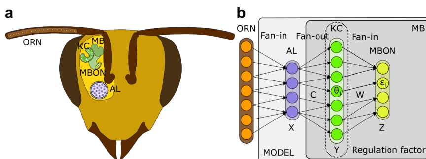
Figura 3.1: Modelo del sistema olfativo del insecto. a Estructura del sistema biológico b Modelo computacional del sistema olfativo basado en una red neuronal de una sola capa oculta
