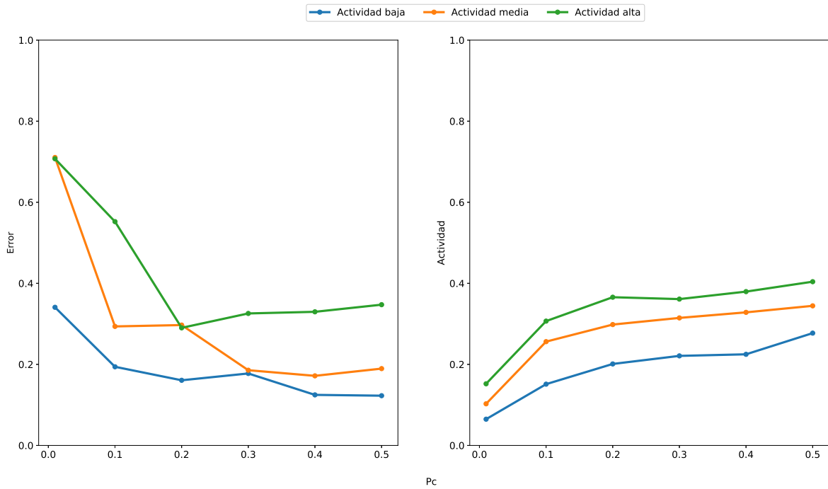
Figura 4.10: Error de clasificación y activación media de las neuronas KCs para las diferentes combinaciones de nivel de actividad con p_c . El modelo se entrena con el conjunto de B_1 y se clasifican los patrones en el conjunto B_2 .
