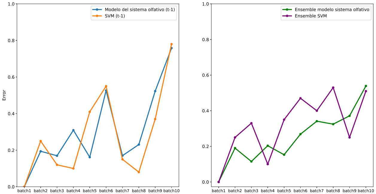
Figura 4.14: Comparación entre los resultados obtenidos clasificando con una SVM o con el modelo de sistema olfativo. La figura de la derecha corresponde a la primera configuración y la figura de la izquierda muestra los resultados para la segunda. Los resultados de clasificación para las SVMs se han obtenido a partir de la Figura 5 de [68].
