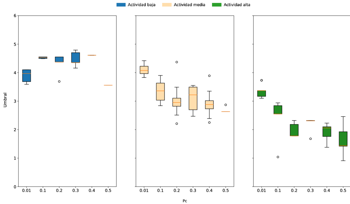
Figura 4.12: Distribuciones del umbral medio en diez simulaciones diferentes para todas las combinaciones de nivel de actividad y p_c .
