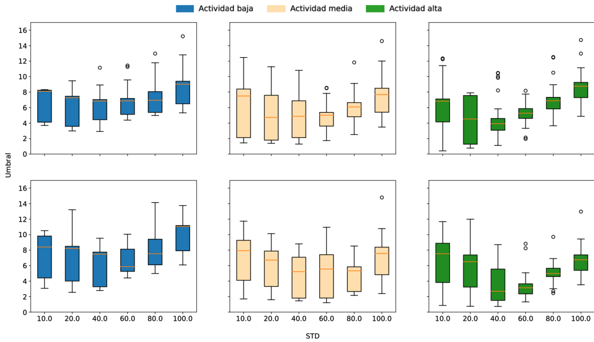
Figura 4.5: Distribución del umbral medio para las diferentes combinaciones de niveles de actividad, complejidad de los patrones con p_c = 0,1 en la línea superior y p_c = 0,4 en la fila inferior. Las distribuciones se han obtenido calculando la media de la distribución de umbrales de cada una de las cinco iteraciones de validación cruzada para diez simulaciones del modelo por cada nivel de complejidad.
