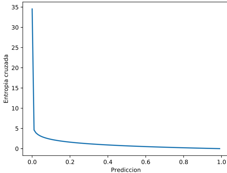
Figura 3.2: Función de entropía cruzada para diferentes valores de predicción teniendo en cuenta que el valor real de la clase es 1.
