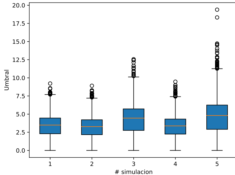
Figura 4.11: Distribuciones de umbrales óptimas para cinco simulaciones con el nivel de actividad bajo y p_c = 0,1 . El modelo se entrena utilizando el conjunto de odorantes 1 y se evalúa clasificando el 2.
