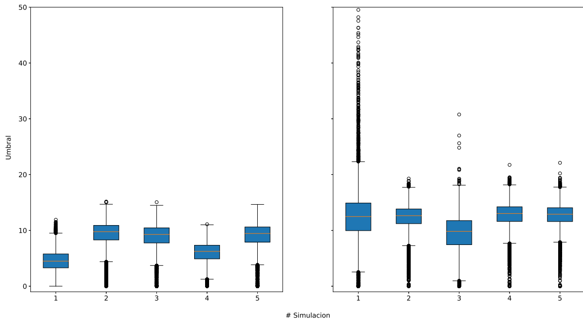
Figura 4.7: Diagramas de cajas para la distribución de umbrales óptimas para actividad baja con p_c = 0,1 a la izquierda y actividad muy baja con p_c = 0,1 a la derecha. Se han elegido estos valores de p_c al ser los que consiguen un error de clasificación más bajo. Se muestran las distribuciones ajustadas para cada una de las cinco iteraciones de validación cruzada en una simulación del modelo.
