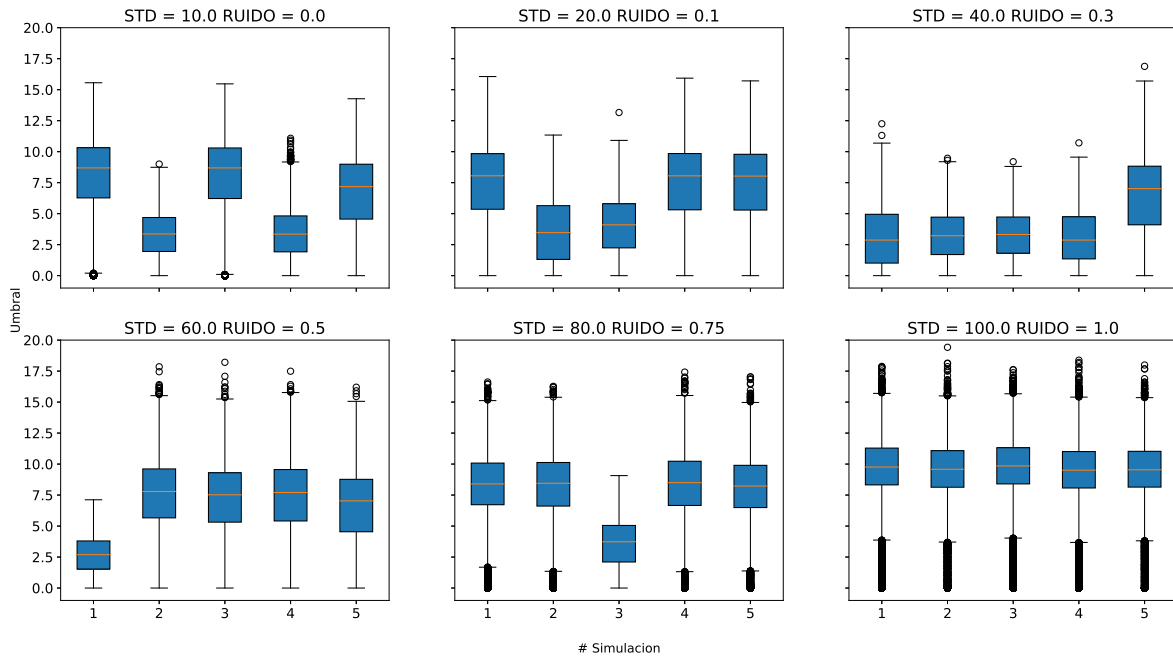
Figura 4.4: Distribución de umbrales neuronales óptima para los diferentes conjuntos de patrones gaussianos y los parámetros p_c = 0,1 y s = 0,1 . Las distribuciones que se muestran se corresponden con cada una de las cinco iteraciones de validación cruzada de una simulación del modelo por cada conjunto de patrones.
