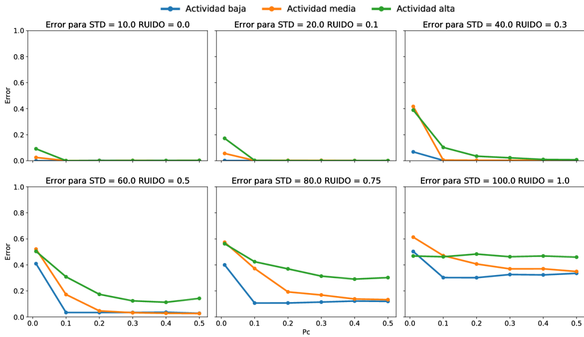
Figura 4.2: Error de clasificación obtenido por el modelo para los diferentes conjuntos de patrones gaussianos de dificultades variables en función del solapamiento entre las clases (consultar Sección 3.3.2). En cada gráfico se presenta el error para los tres niveles de actividad considerados en combinación con diferentes valores de p_c en el intervalo [0,01, 0,5] .
