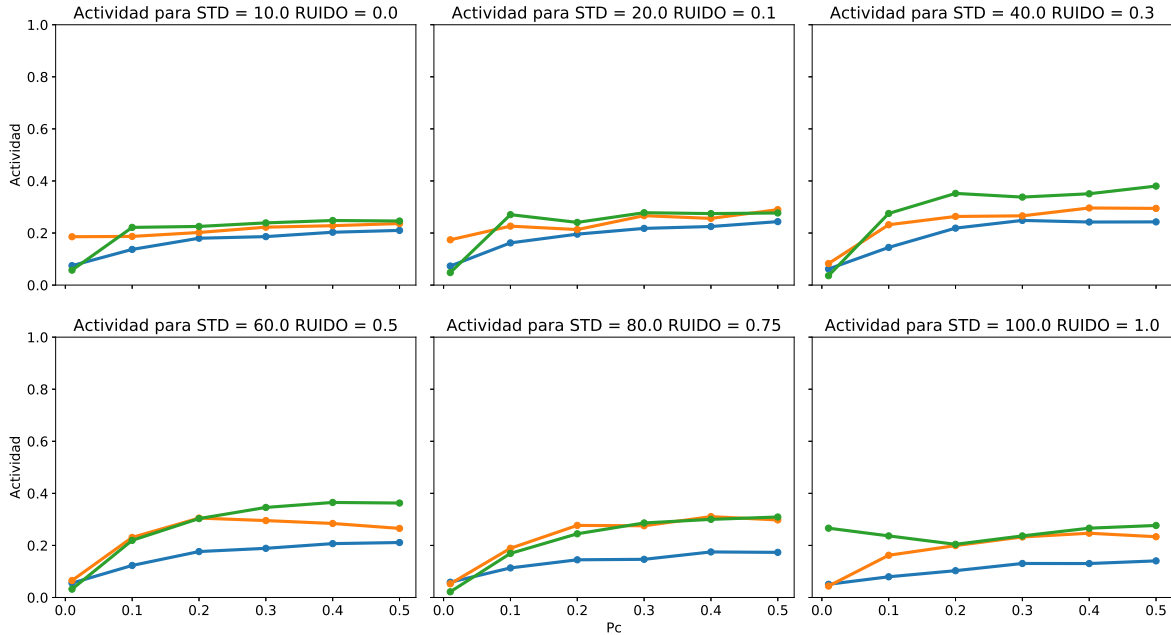
Figura 4.3: Nivel de activación medio de las neuronas KCs para los diferentes conjuntos de patrones gaussianos de dificultades variables en función del solapamiento entre las clases (consultar Sección 3.3.2). En cada gráfico se muestra el nivel de activación para los tres niveles de actividad utilizados y los diferentes valores de p_c en el intervalo [0,01, 0,5] .
