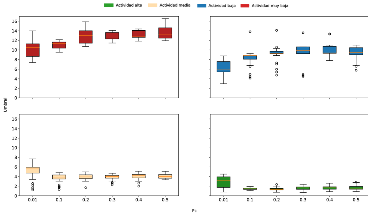
Figura 4.8: Diagrama de la distribución del umbral neuronal medio para los patrones MNIST con los diferentes niveles de actividad y valores de p_c . Los resultados se han obtenido mediante 10 simulaciones por cada combinación con validación cruzada con 5 iteraciones.
