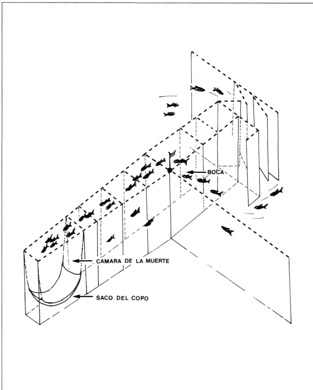
Figura 8: Reconstrucción ideal de la disposición de una almadraba. (Dibujo propio basado en ilustración de Artero, 1974, 30)
