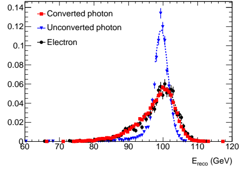
(d) E = 100\text{GeV}
