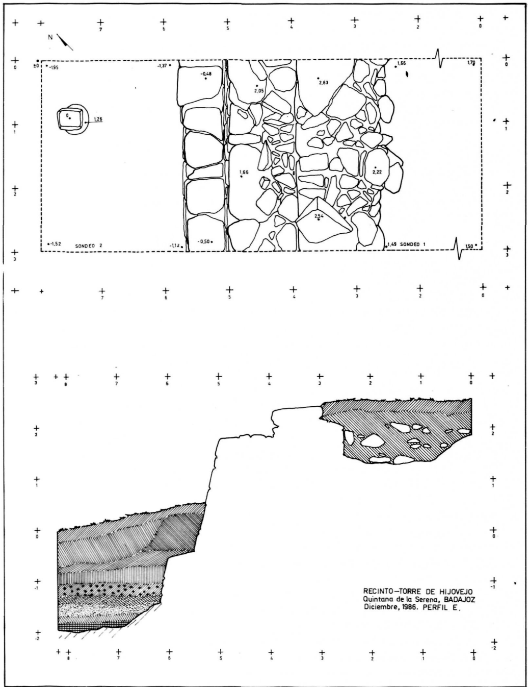
Figura 8. Hijojejo, 1986: planta y perfil de los sondes 1 y 2.
