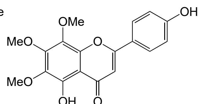
Xanthomicrol
