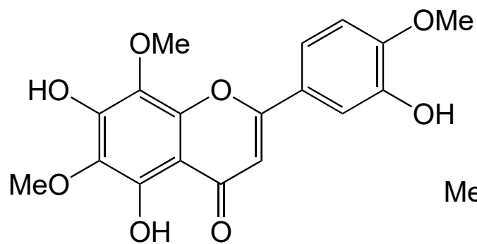
Acerosin
