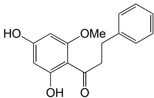
Cardamonin
