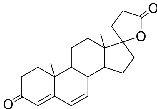
Canrenone
