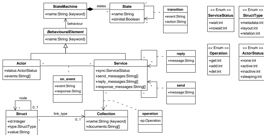
Fig. 1. The VisMODLE Meta-model.
