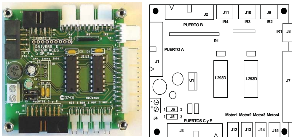
Fig.3: Foto de la Tarjeta GP_Bot_Ifaz y su distribución de componentes.
