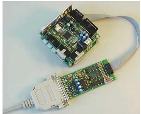
Fig.1: Tarjetas GP_Bot y GP_Mon.
