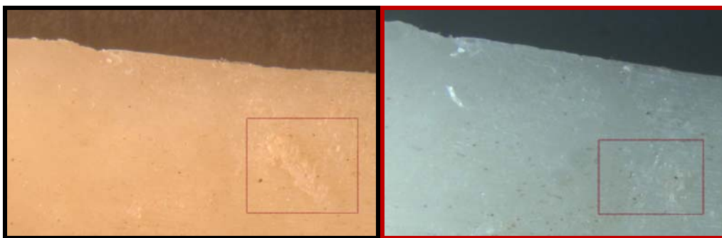
Figura 10 .Pieza previa a la experiencia (img. izq.) y pieza tras la experiencia (img. drch.)
