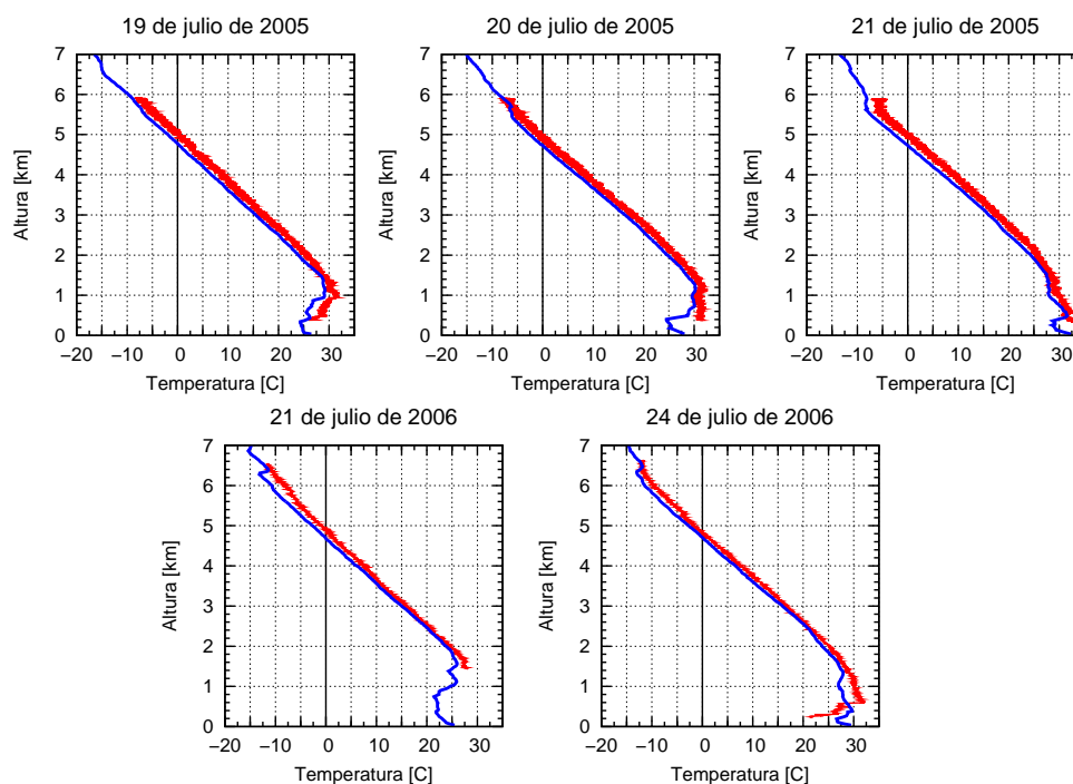
Figura 5.12: Comparación de perfiles verticales de temperatura de los ozonsondeos (azul) y de la plataforma aérea (rojo)
