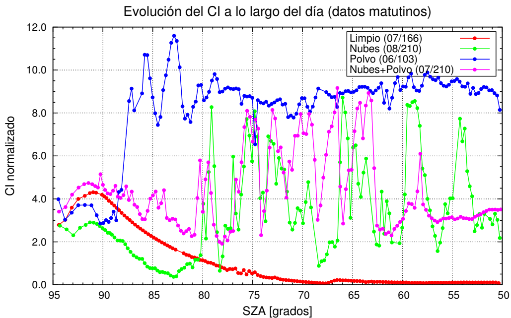
Figura 3.7: Valores observados del CI a lo largo de la mañana bajo distintos escenarios
