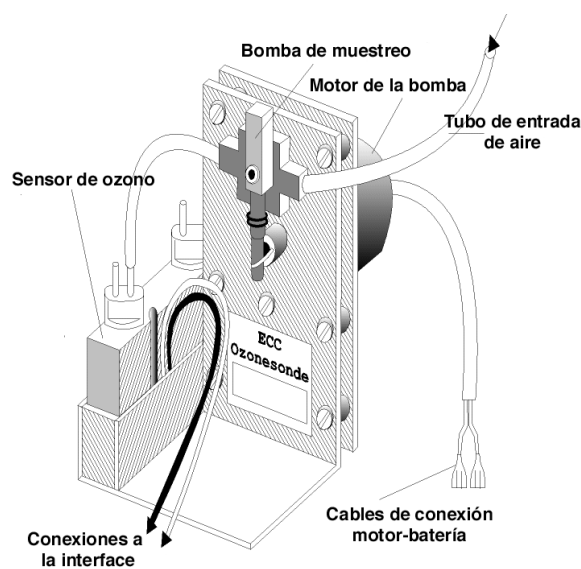
Figura 4.4: Esquema de una ozonosonda y las partes que la componen
