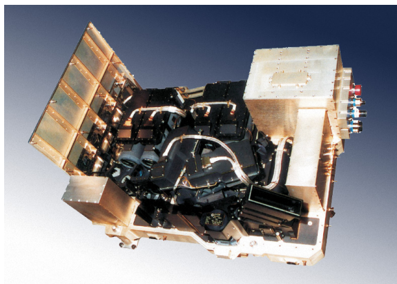
Figura 4.10: Espectrómetro GOME 2
