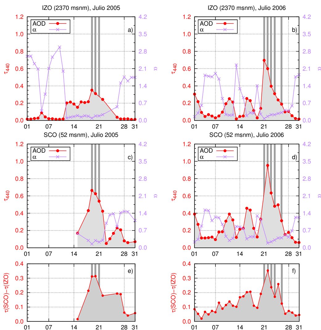
Figura 5.6: Evolución del espesor óptico de aerosoles y del exponente de Ångstrom en Izaña (paneles a,b) y en Santa Cruz de Tenerife (c,d) y diferencias entre ambas estaciones (e,f) durante los meses de julio de 2005 y 2006. Las barras grises indican los días en que se realizaron los vuelos.
