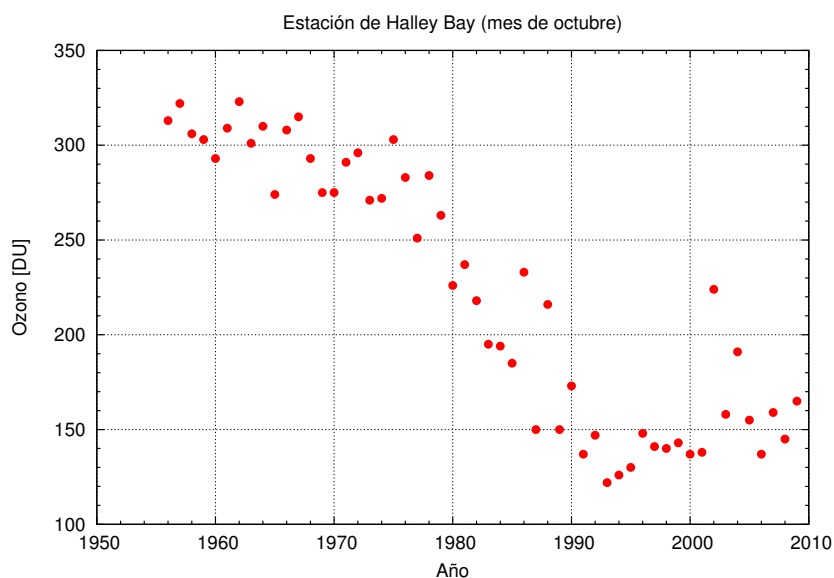
Figura 2.5: Valores medios de la columna total de ozono en la estación de Halley Bay ( 75.6 \text{ S} , 34.6 \text{ W} ) durante el mes de octubre. Elaboración propia a partir de datos del British Antarctic Survey (BAS).
