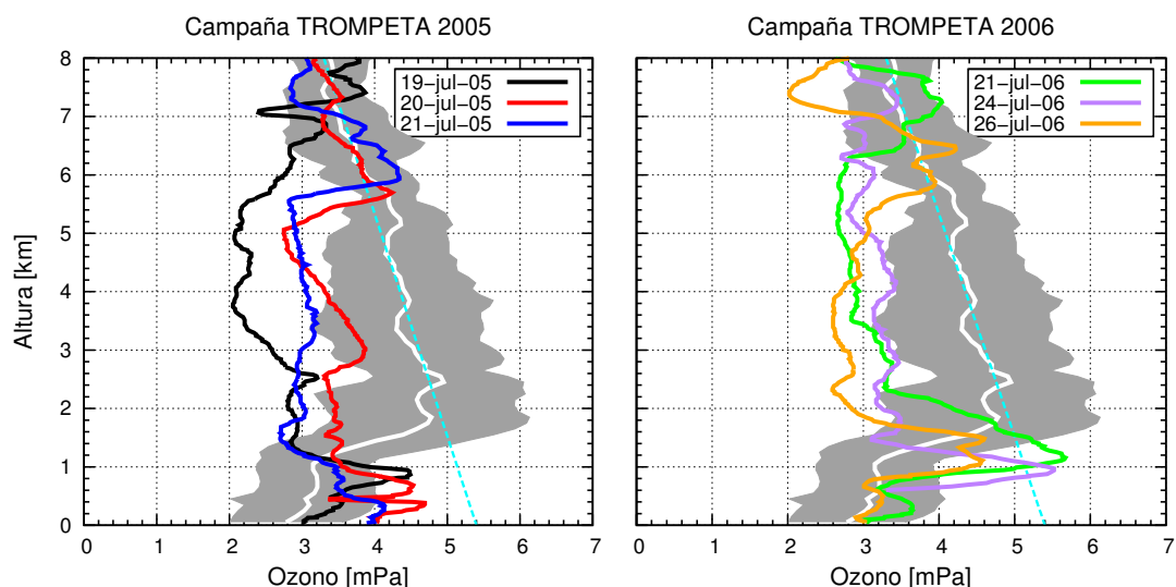
Figura 5.10: Ozonosondeos realizados durante las campañas TROPETA y perfil vertical medio de ozono de las islas Canarias durante el mes de julio. La zona sombreada corresponde a una desviación estándar.
